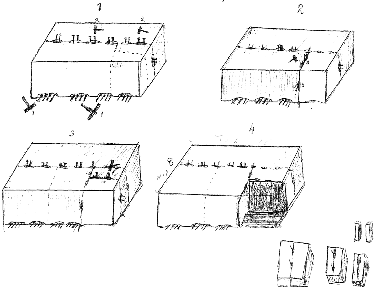
Disinn magħmul minn Innocenzo Camilleri fl-1976, biex ifiehem il-proċess tal-qtugħ tal-ġebel bl-ispanjar sakemm fl-aħhar tasal biex ikollok kantun.
